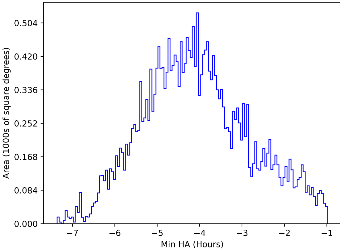
too_elab_r16_d3_ugrizy_v3.4_10yrs All sky i band: Min HA
