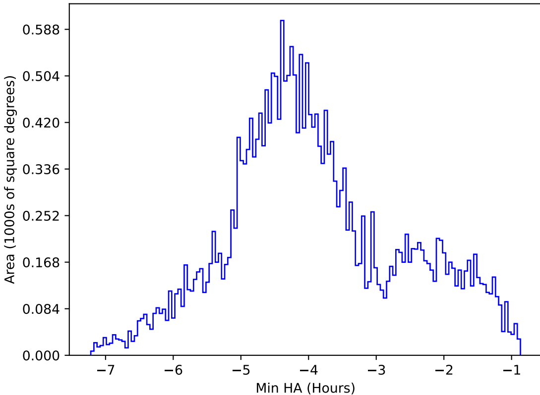
too_elab_r16_d3_ugrizy_v3.4_10yrs All sky g band: Min HA
