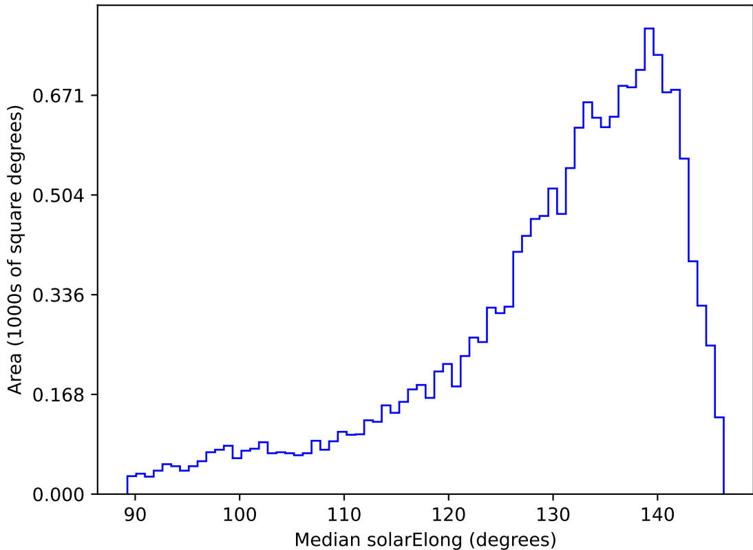
too_elab_r16_d3_ugrizy_v3.4_10yrs WFD y band: Median solarElong
