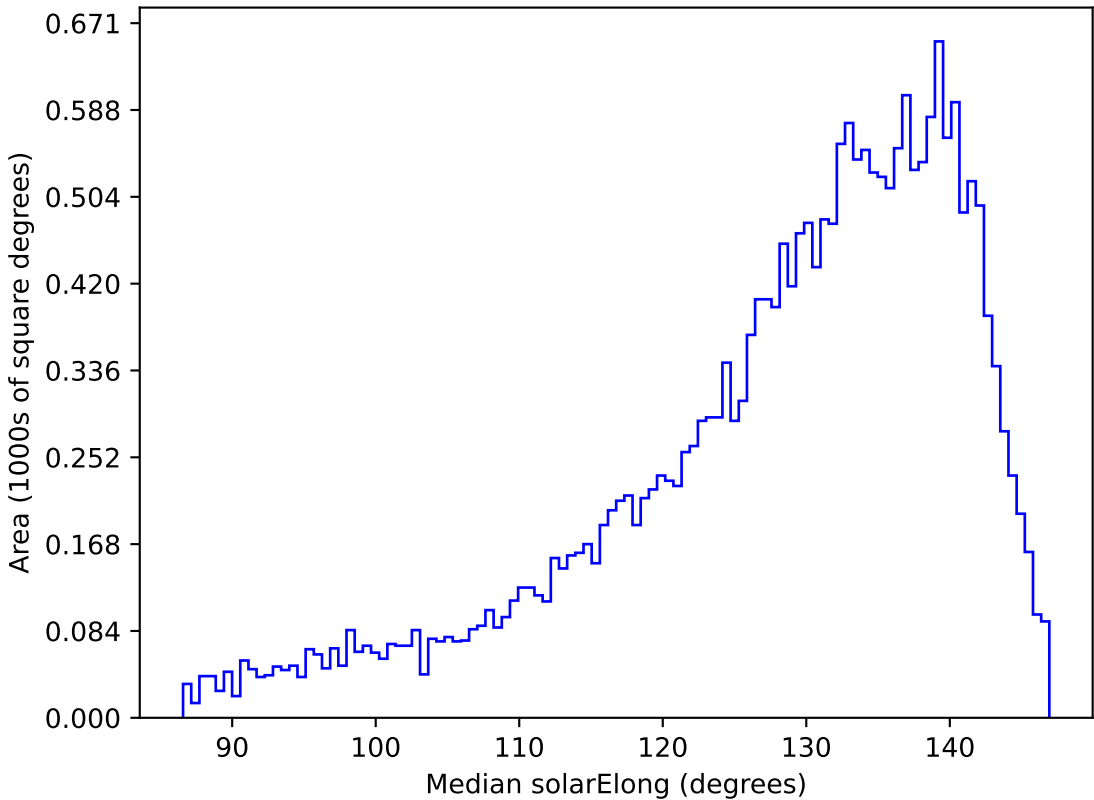
too_elab_r16_d3_ugrizy_v3.4_10yrs All sky y band: Median solarElong
