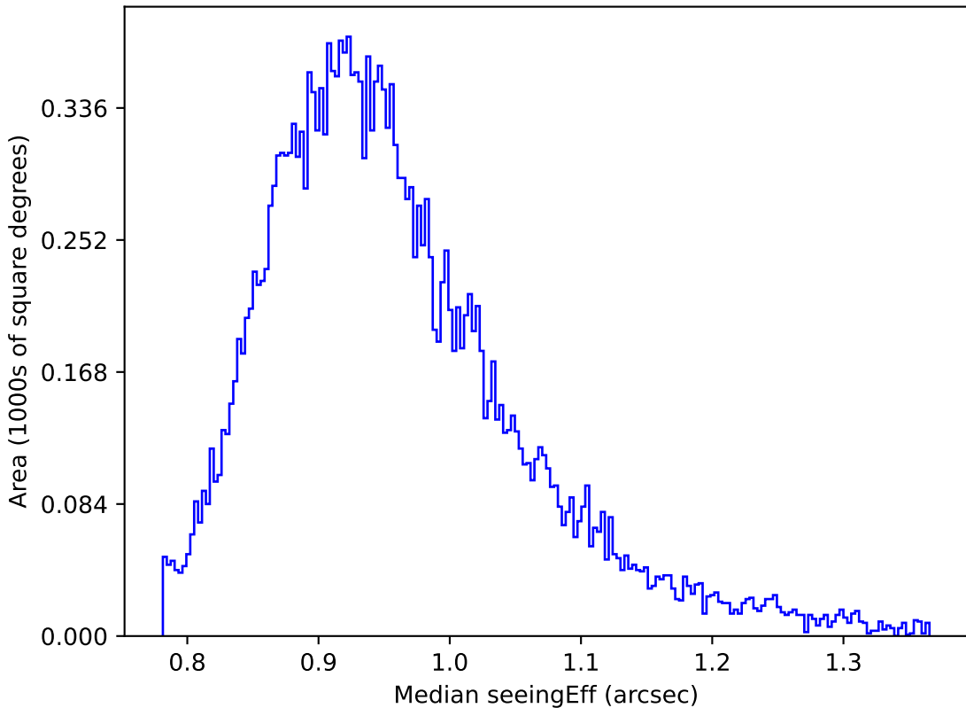
too_elab_r16_d3_ugrizy_v3.4_10yrs Yr 1 y band: Median seeingEff
