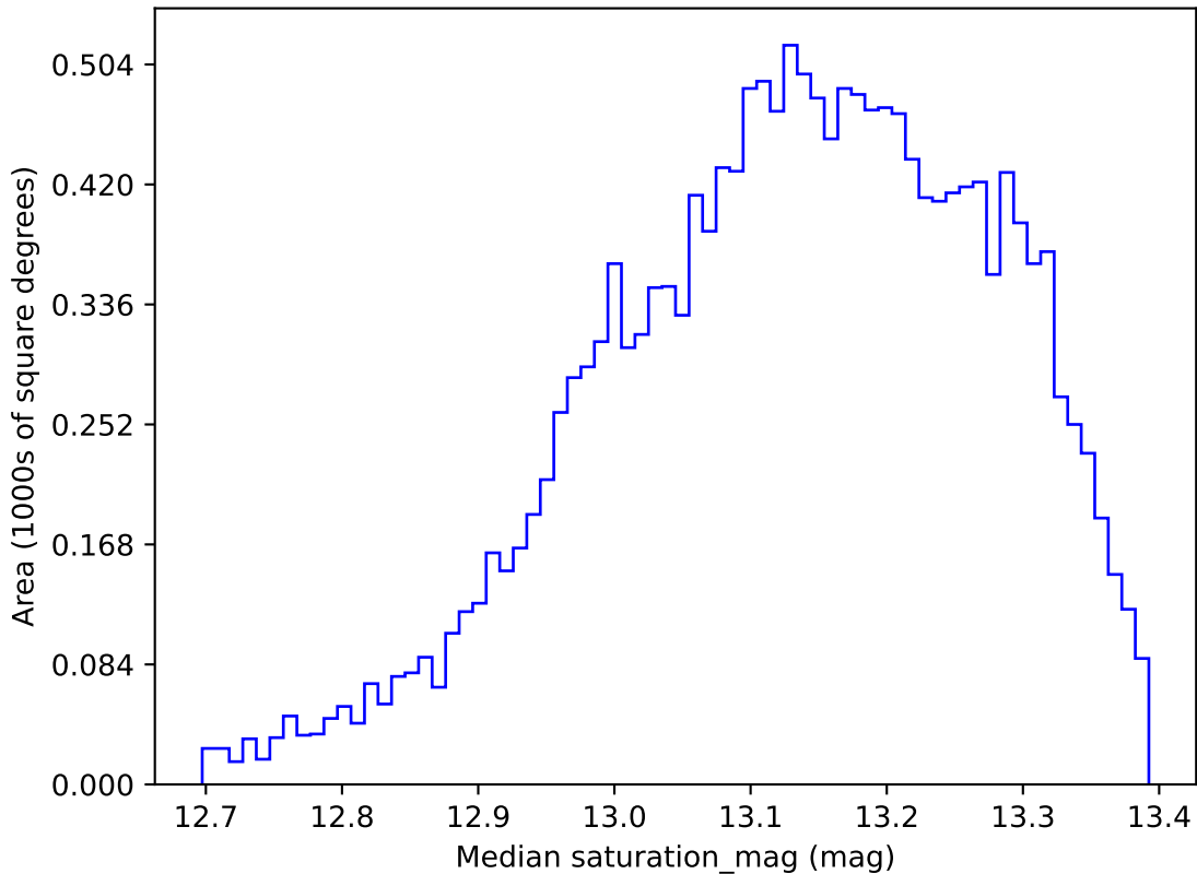
too_elab_r16_d3_ugrizy_v3.4_10yrs WFD y band: Median saturation_mag
