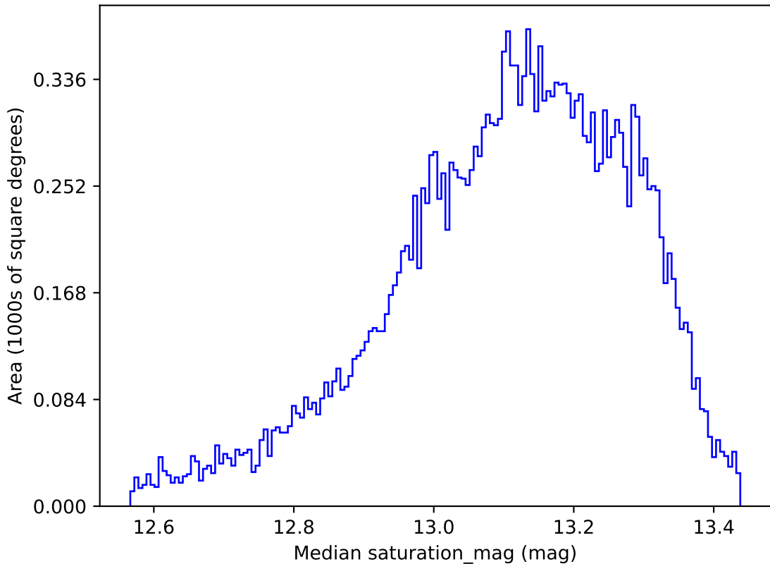
too_elab_r16_d3_ugrizy_v3.4_10yrs All sky y band: Median saturation_mag
