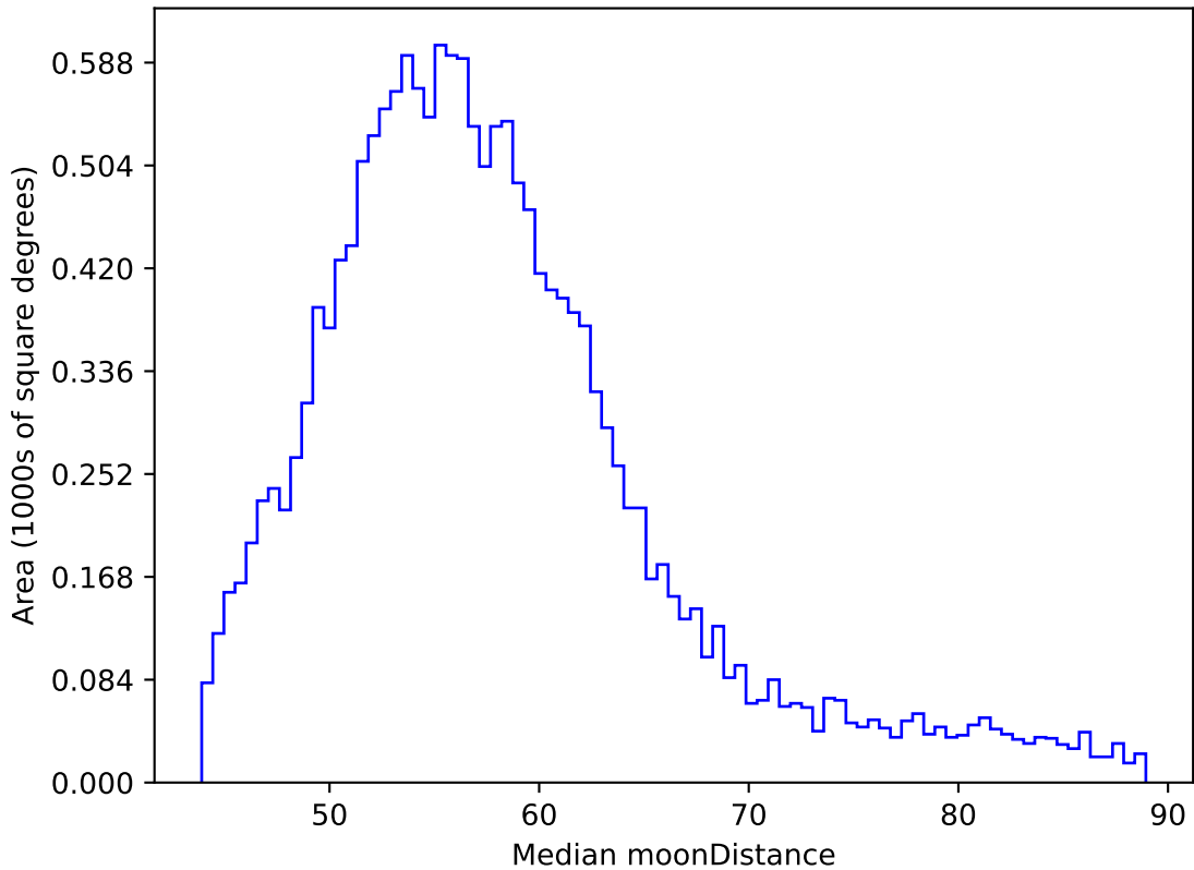
too_elab_r16_d3_ugrizy_v3.4_10yrs WFD y band: Median moonDistance
