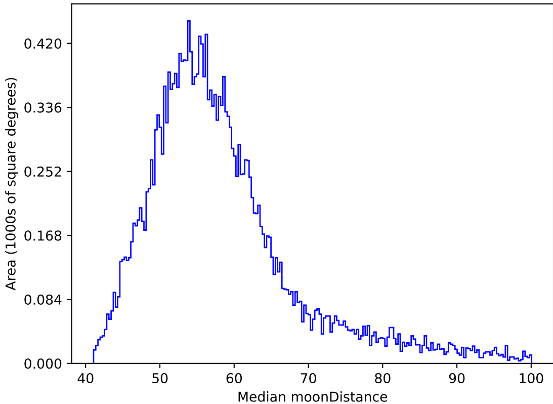
too_elab_r16_d3_ugrizy_v3.4_10yrs All sky y band: Median moonDistance
