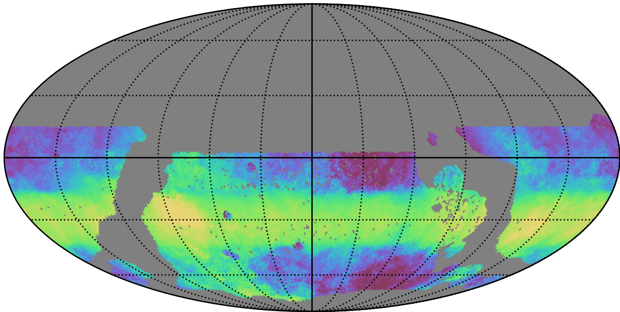
too_elab_r16_d3_ugrizy_v3.4_10yrs WFD y band: Median HA
