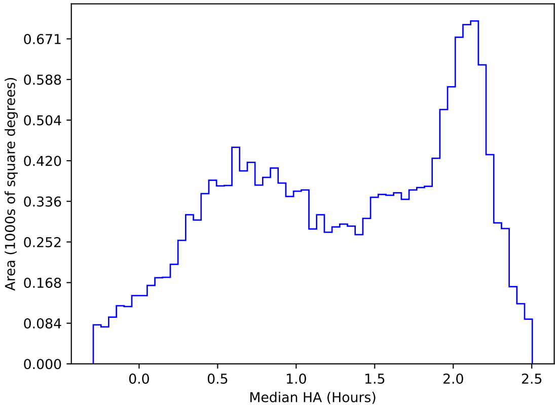
too_elab_r16_d3_ugrizy_v3.4_10yrs WFD y band: Median HA
