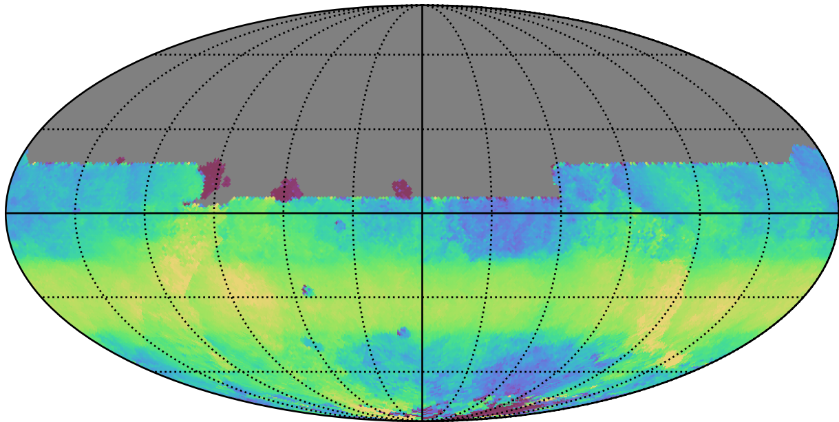
too_elab_r16_d3_ugrizy_v3.4_10yrs All sky y band: Median HA
