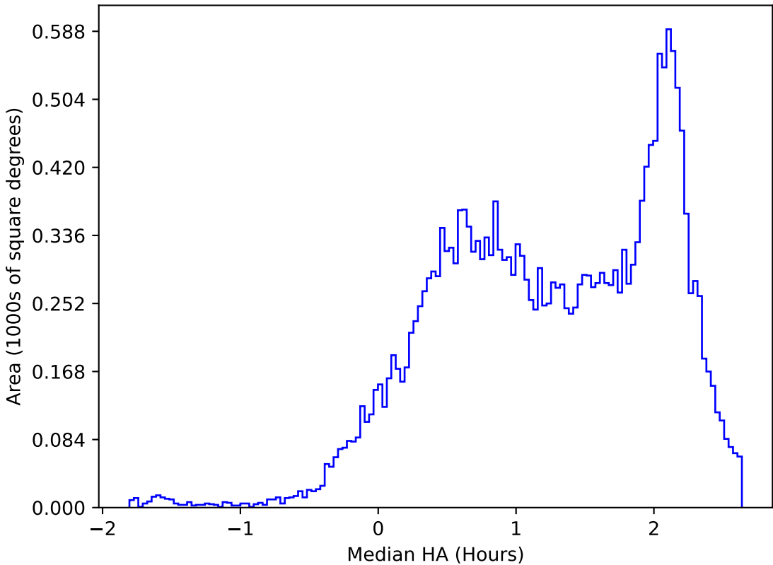
too_elab_r16_d3_ugrizy_v3.4_10yrs All sky y band: Median HA
