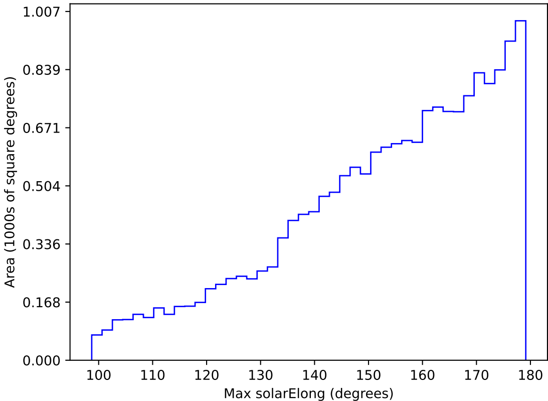
too_elab_r16_d3_ugrizy_v3.4_10yrs WFD y band: Max solarElong
