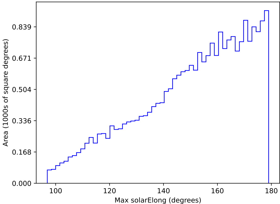
too_elab_r16_d3_ugrizy_v3.4_10yrs All sky y band: Max solarElong
