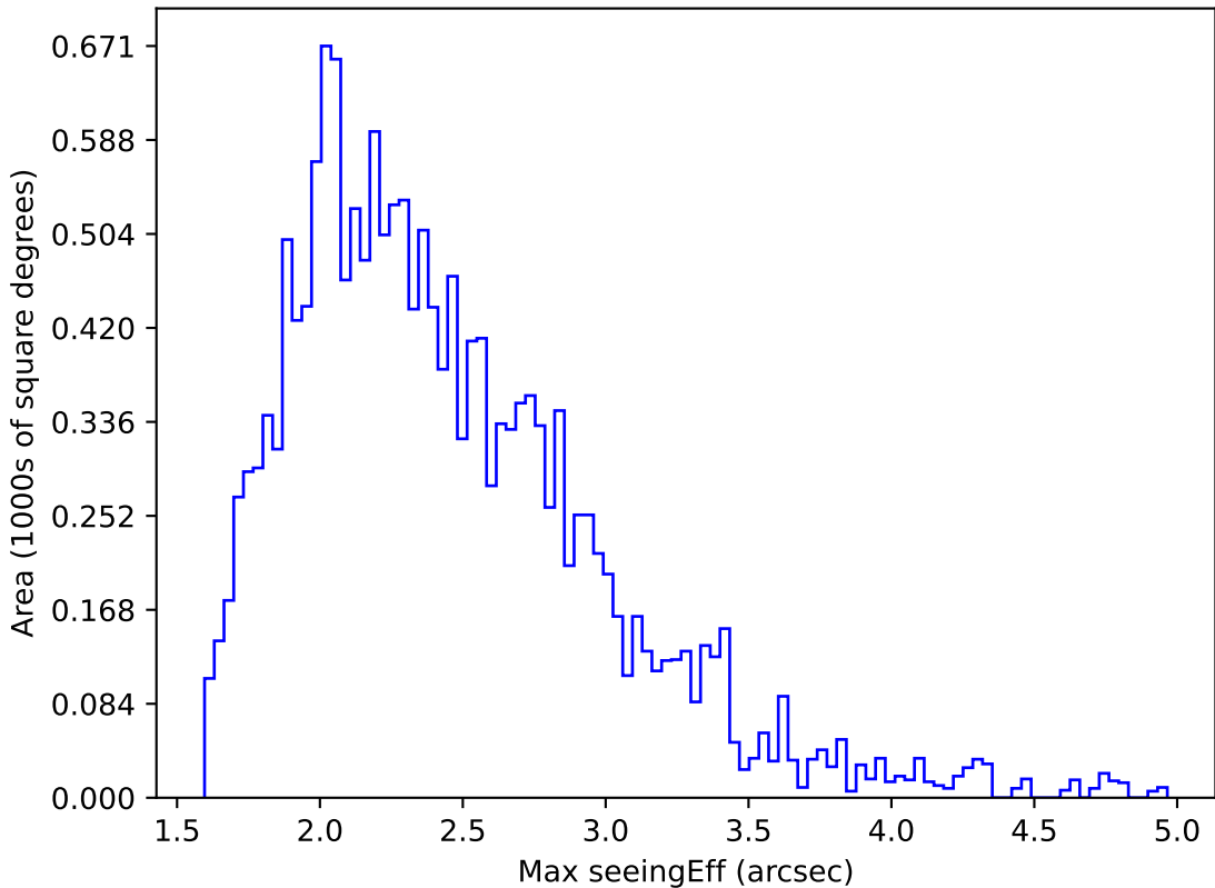
too_elab_r16_d3_ugrizy_v3.4_10yrs WFD y band: Max seeingEff
