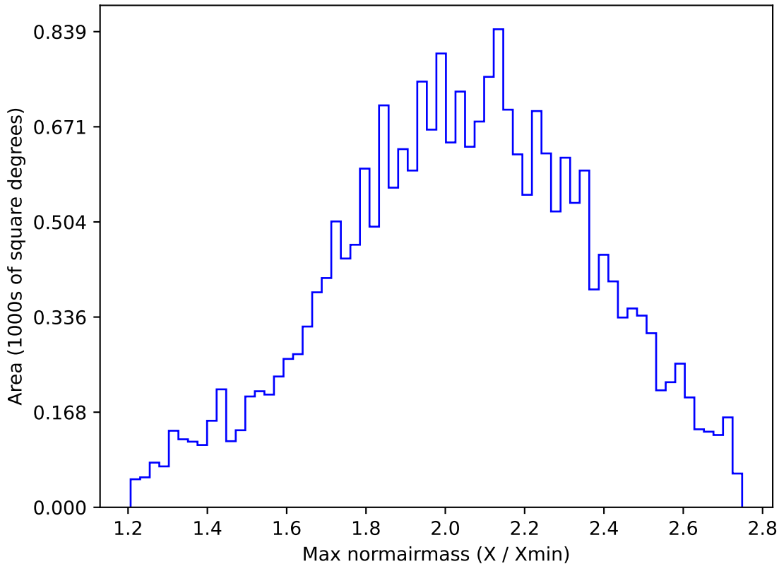
too_elab_r16_d3_ugrizy_v3.4_10yrs All sky y band: Max normairmass
