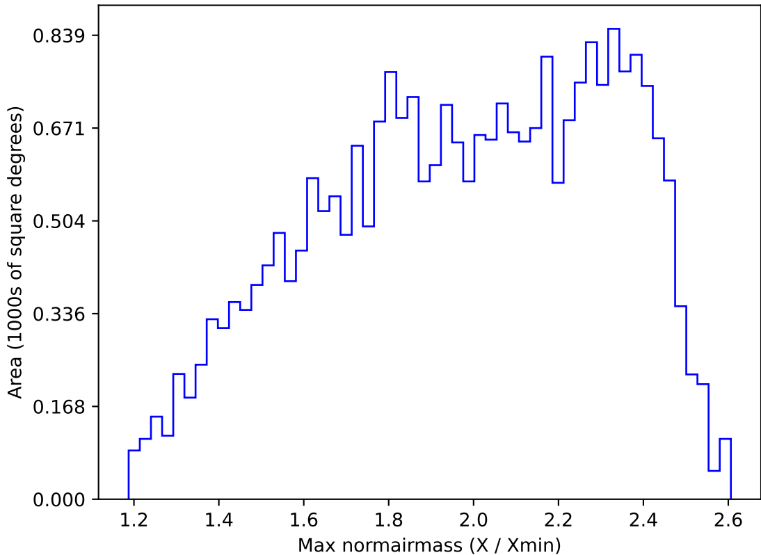
too_elab_r16_d3_ugrizy_v3.4_10yrs All sky r band: Max normairmass
