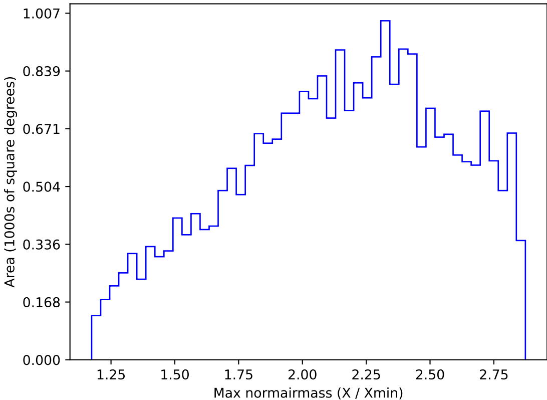
too_elab_r16_d3_ugrizy_v3.4_10yrs All sky i band: Max normairmass
