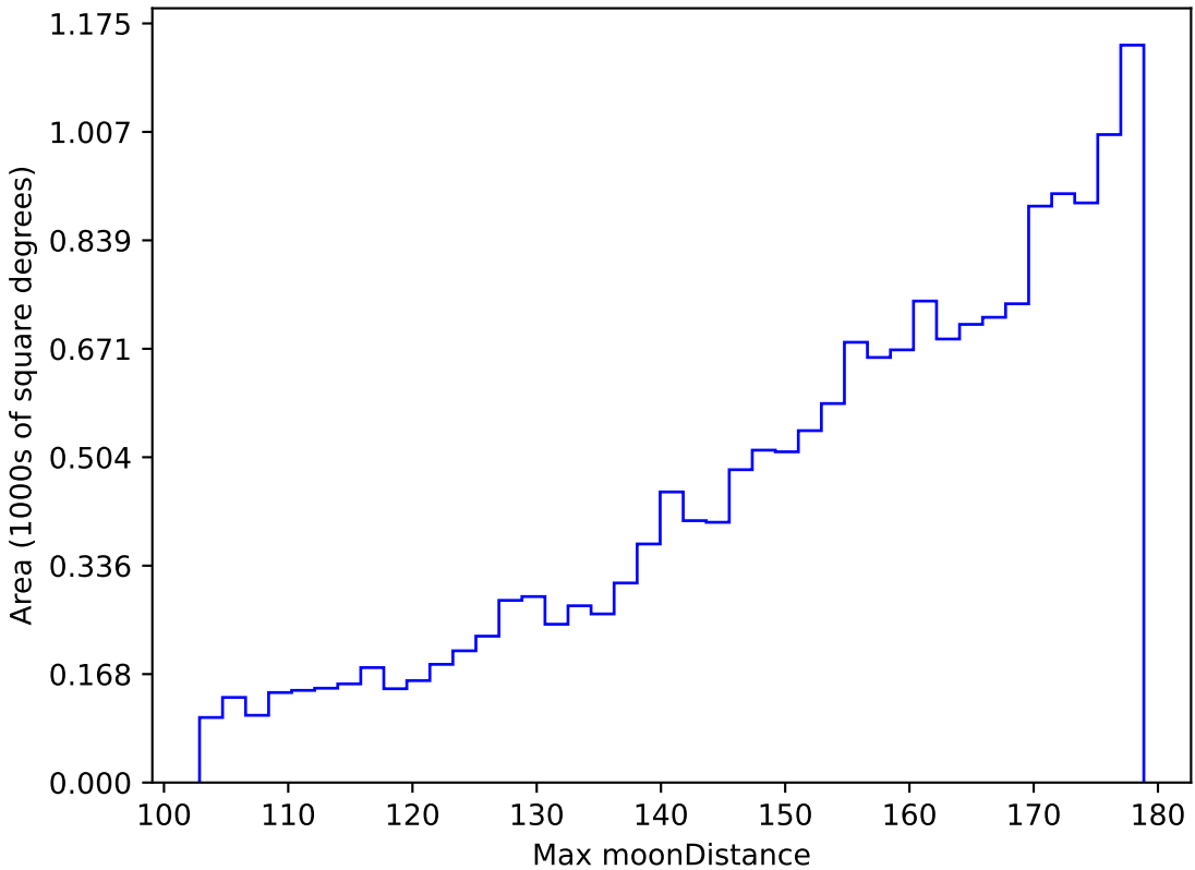
too_elab_r16_d3_ugrizy_v3.4_10yrs WFD z band: Max moonDistance
