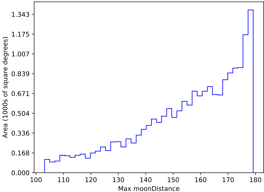
too_elab_r16_d3_ugrizy_v3.4_10yrs WFD i band: Max moonDistance
