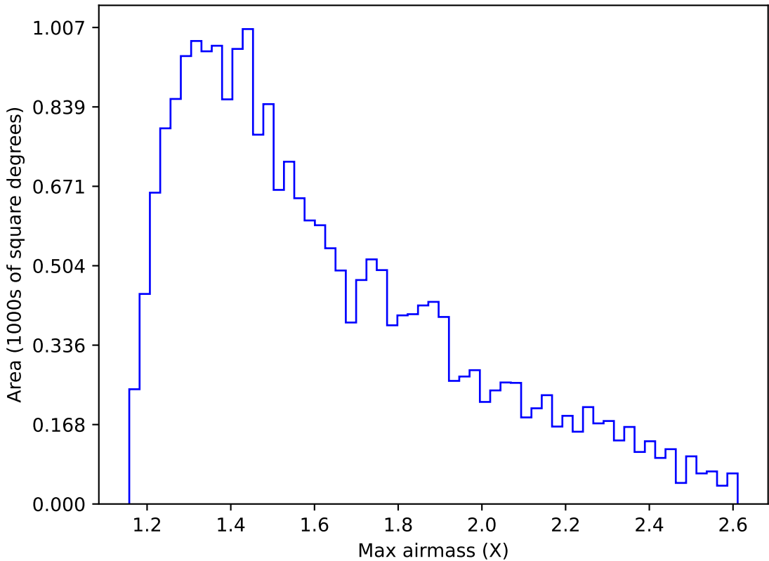
too_elab_r16_d3_ugrizy_v3.4_10yrs Yr 1 y band: Max airmass
