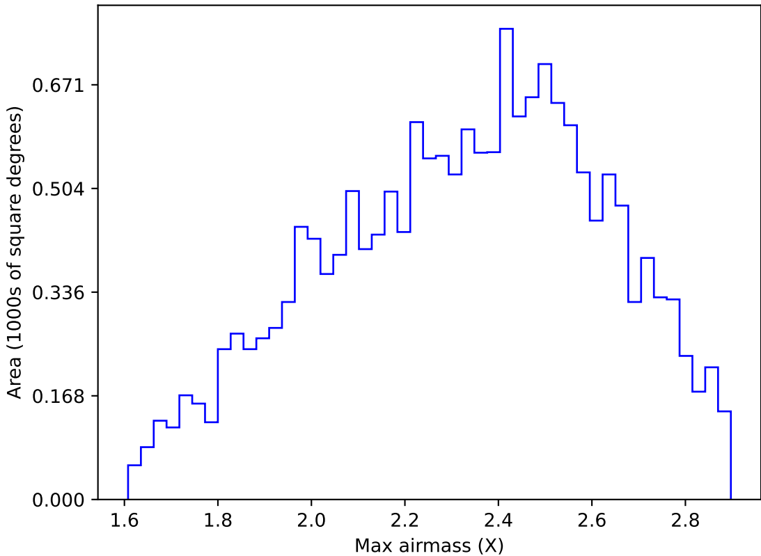
too_elab_r16_d3_ugrizy_v3.4_10yrs WFD y band: Max airmass
