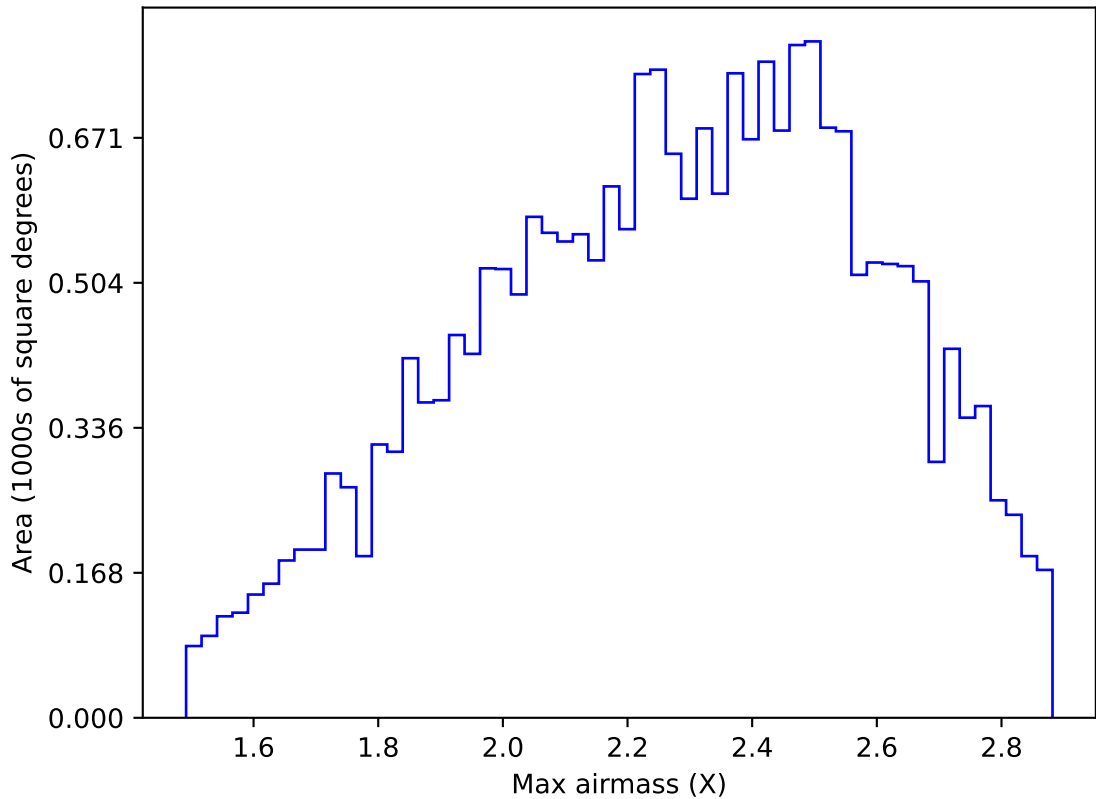
too_elab_r16_d3_ugrizy_v3.4_10yrs All sky y band: Max airmass
