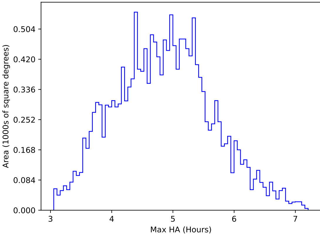
too_elab_r16_d3_ugrizy_v3.4_10yrs WFD z band: Max HA
