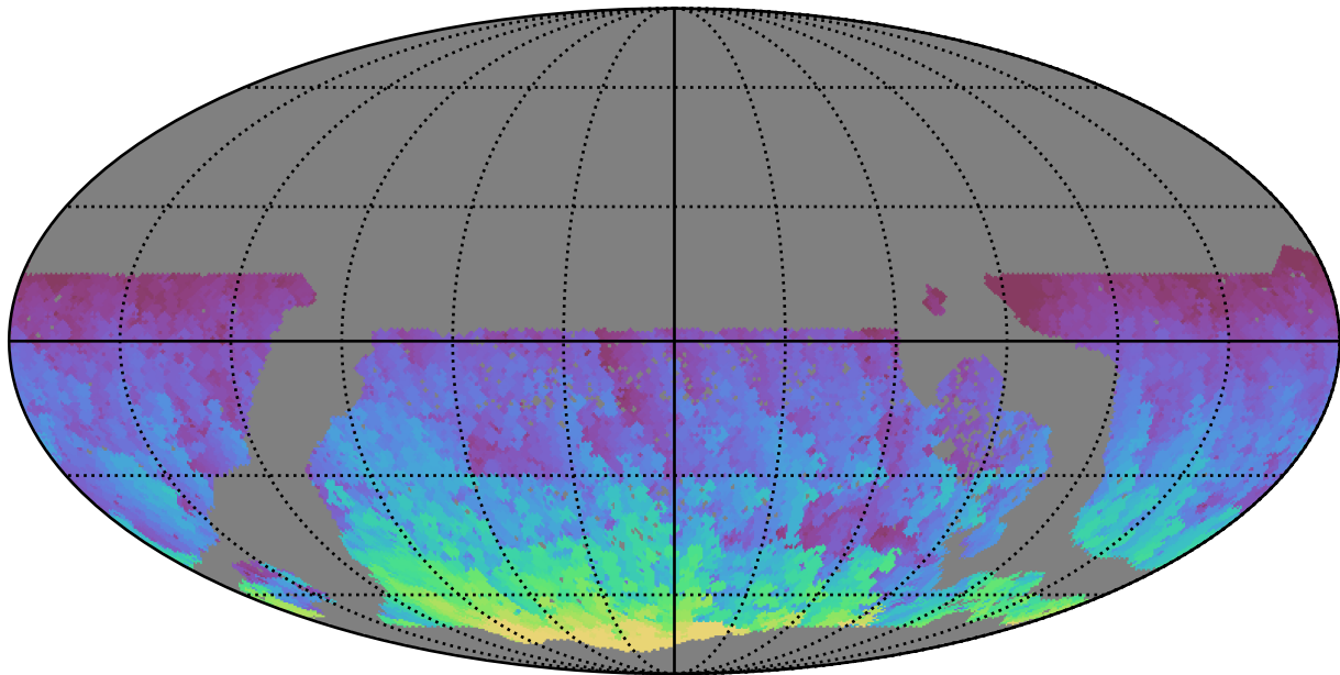
too_elab_r16_d3_ugrizy_v3.4_10yrs WFD y band: Max HA
