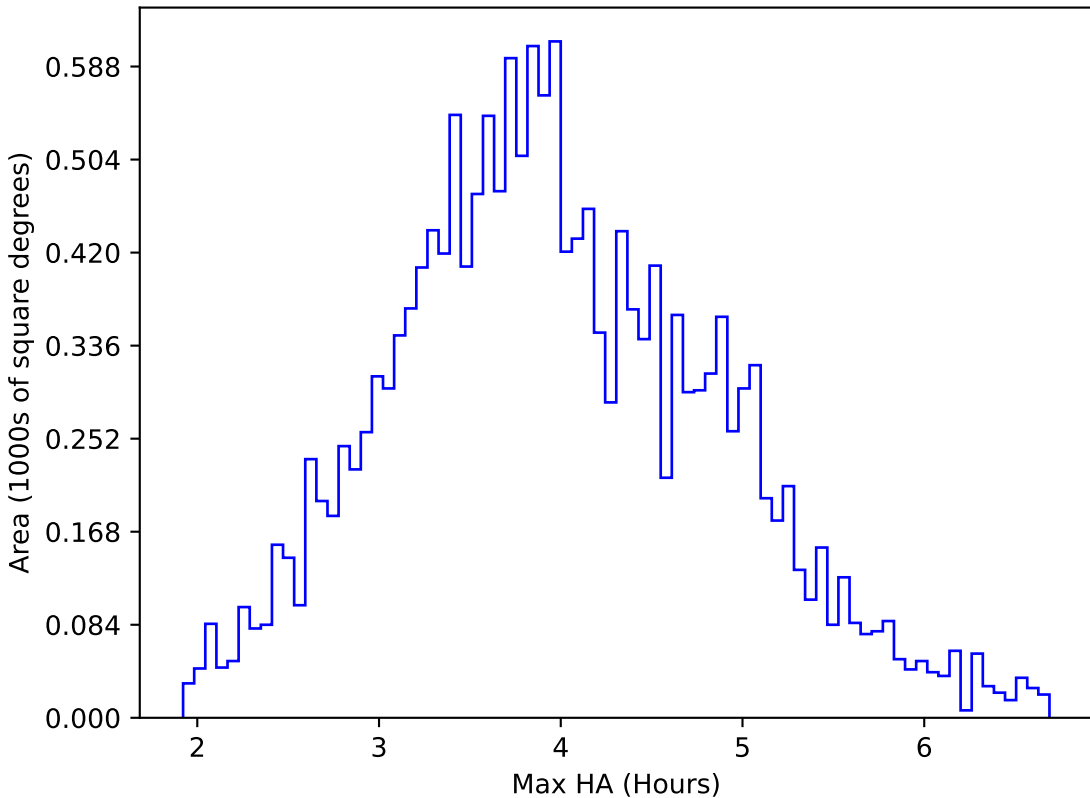
too_elab_r16_d3_ugrizy_v3.4_10yrs WFD u band: Max HA
