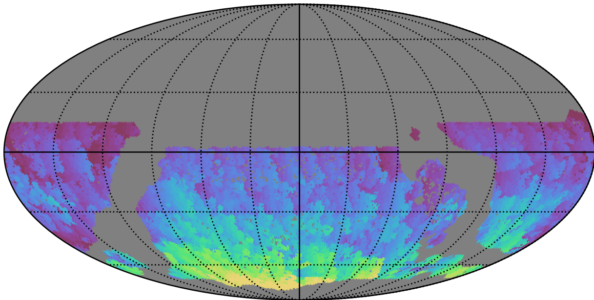
too_elab_r16_d3_ugrizy_v3.4_10yrs WFD r band: Max HA
