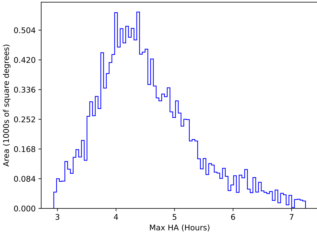
too_elab_r16_d3_ugrizy_v3.4_10yrs WFD r band: Max HA
