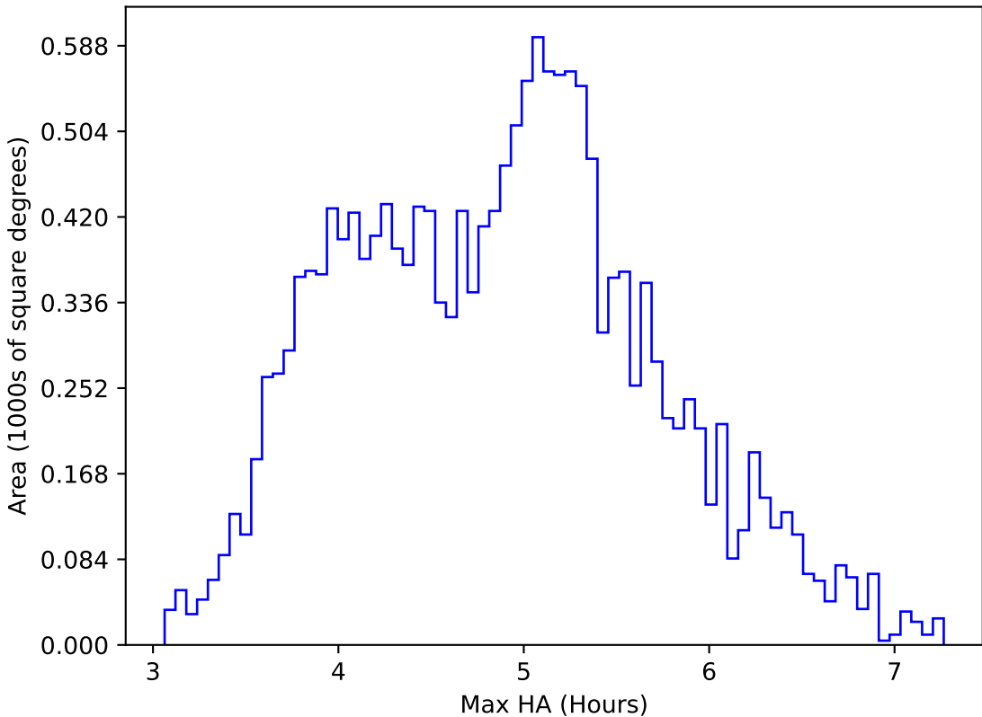
too_elab_r16_d3_ugrizy_v3.4_10yrs WFD i band: Max HA
