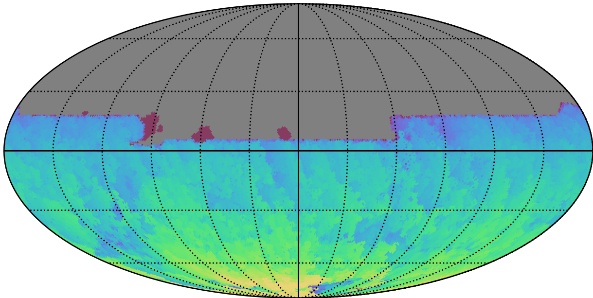
too_elab_r16_d3_ugrizy_v3.4_10yrs All sky y band: Max HA
