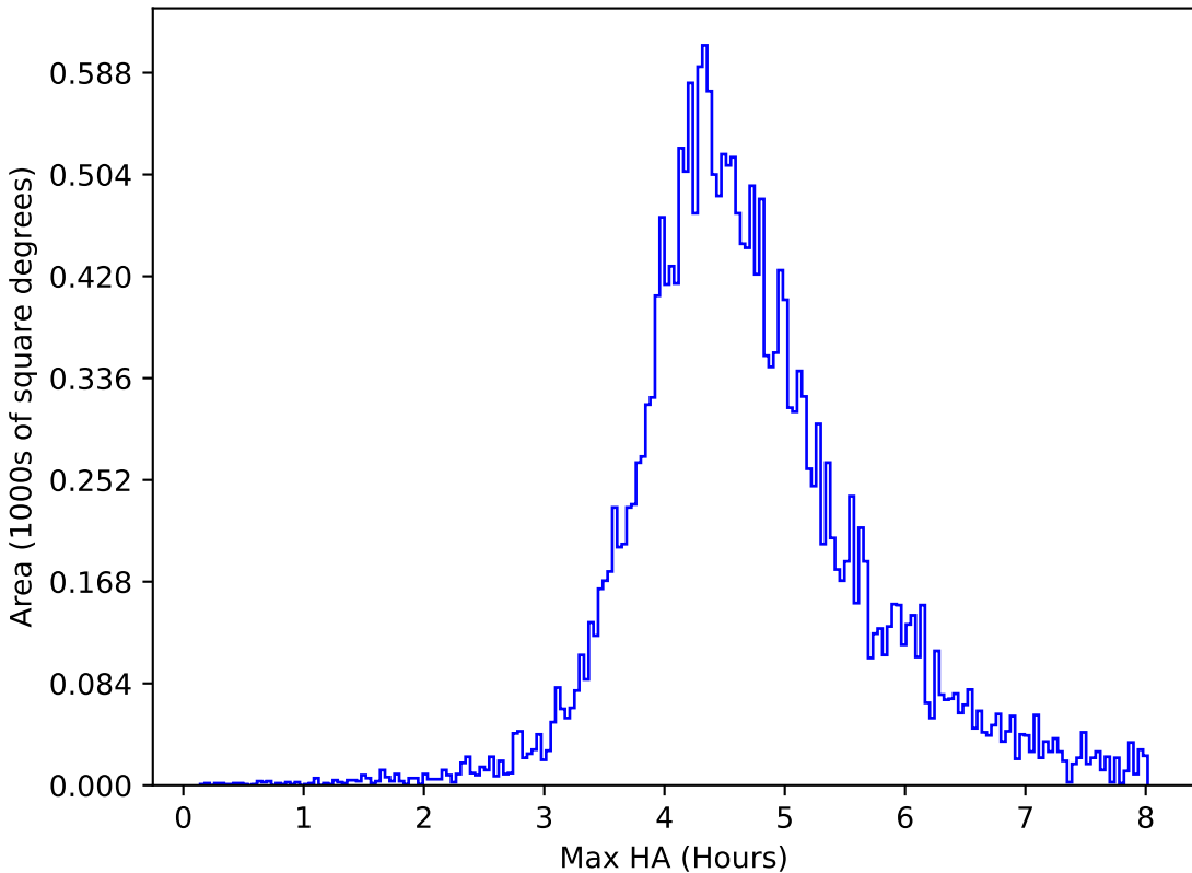
too_elab_r16_d3_ugrizy_v3.4_10yrs All sky y band: Max HA
