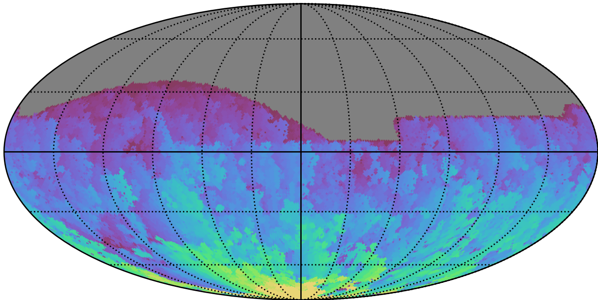
too_elab_r16_d3_ugrizy_v3.4_10yrs All sky g band: Max HA
