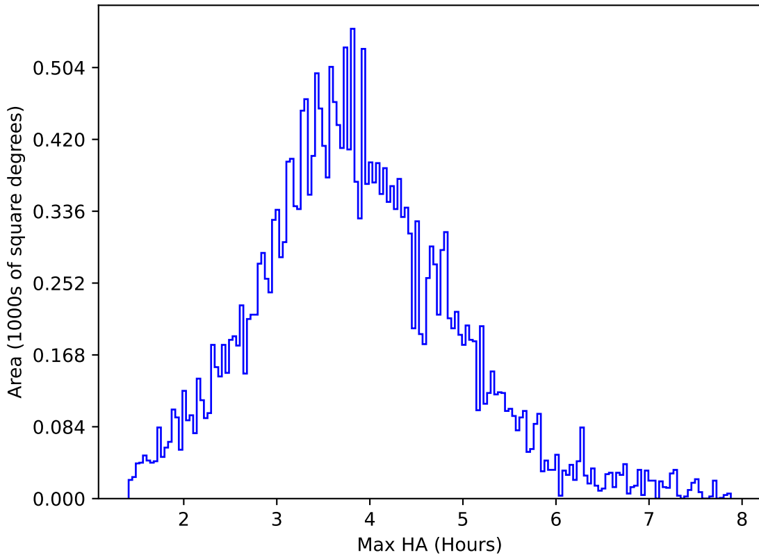
too_elab_r16_d3_ugrizy_v3.4_10yrs All sky g band: Max HA
