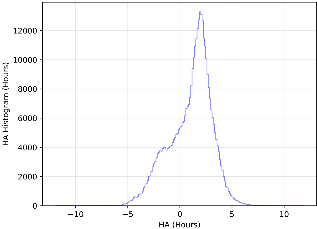
too_elab_r16_d3_ugrizy_v3.4_10yrs WFD y band: HA Histogram
