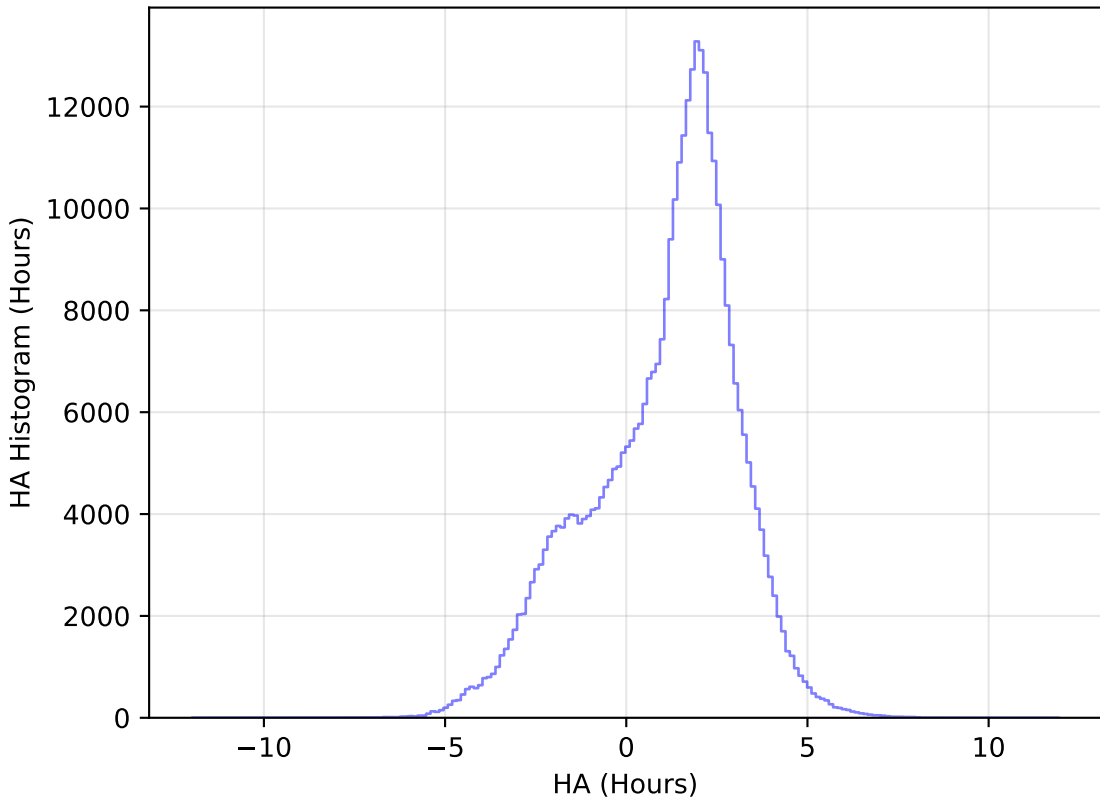
too_elab_r16_d3_ugrizy_v3.4_10yrs All sky y band: HA Histogram
