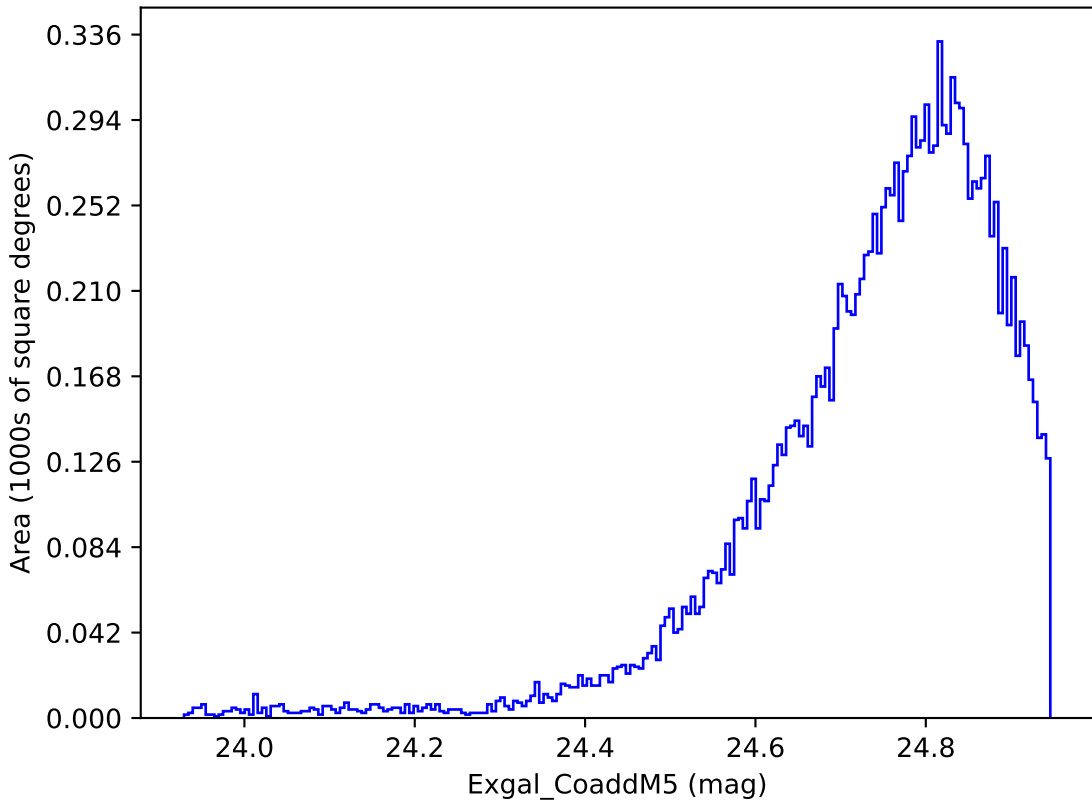
too_elab_r16_d3_ugrizy_v3.4_10yrs WFD y band: Exgal_CoaddM5
