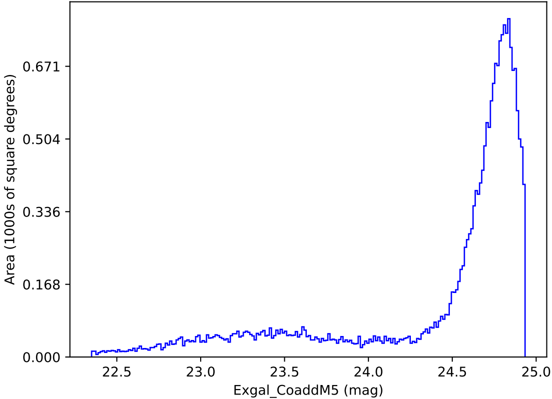
too_elab_r16_d3_ugrizy_v3.4_10yrs All sky y band: Exgal_CoaddM5
