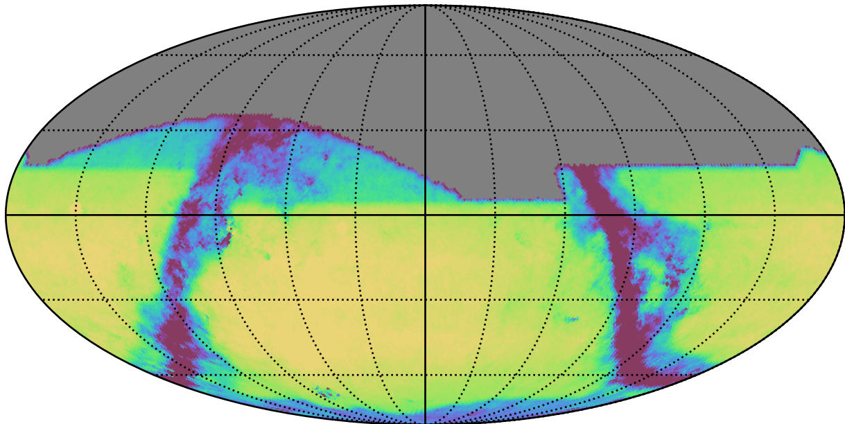
too_elab_r16_d3_ugrizy_v3.4_10yrs All sky i band: Exgal_CoaddM5
