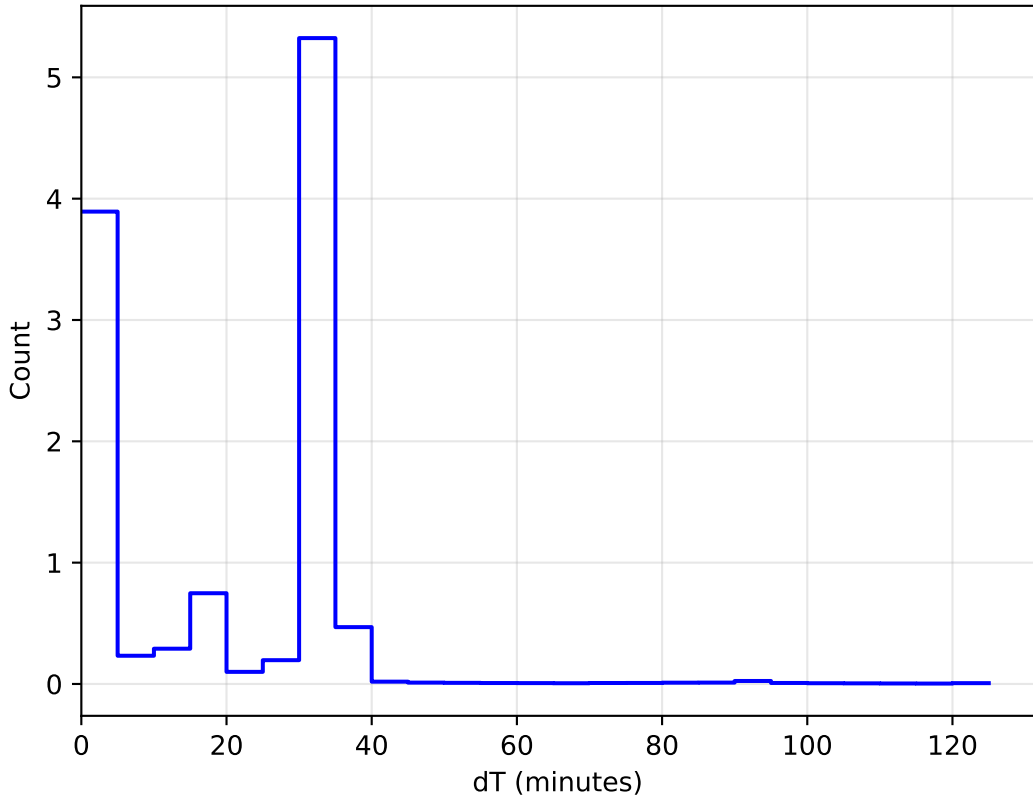
too_elab_r16_d3_ugrizy_v3.4_10yrs WFD: DeltaT Histogram 1e6
