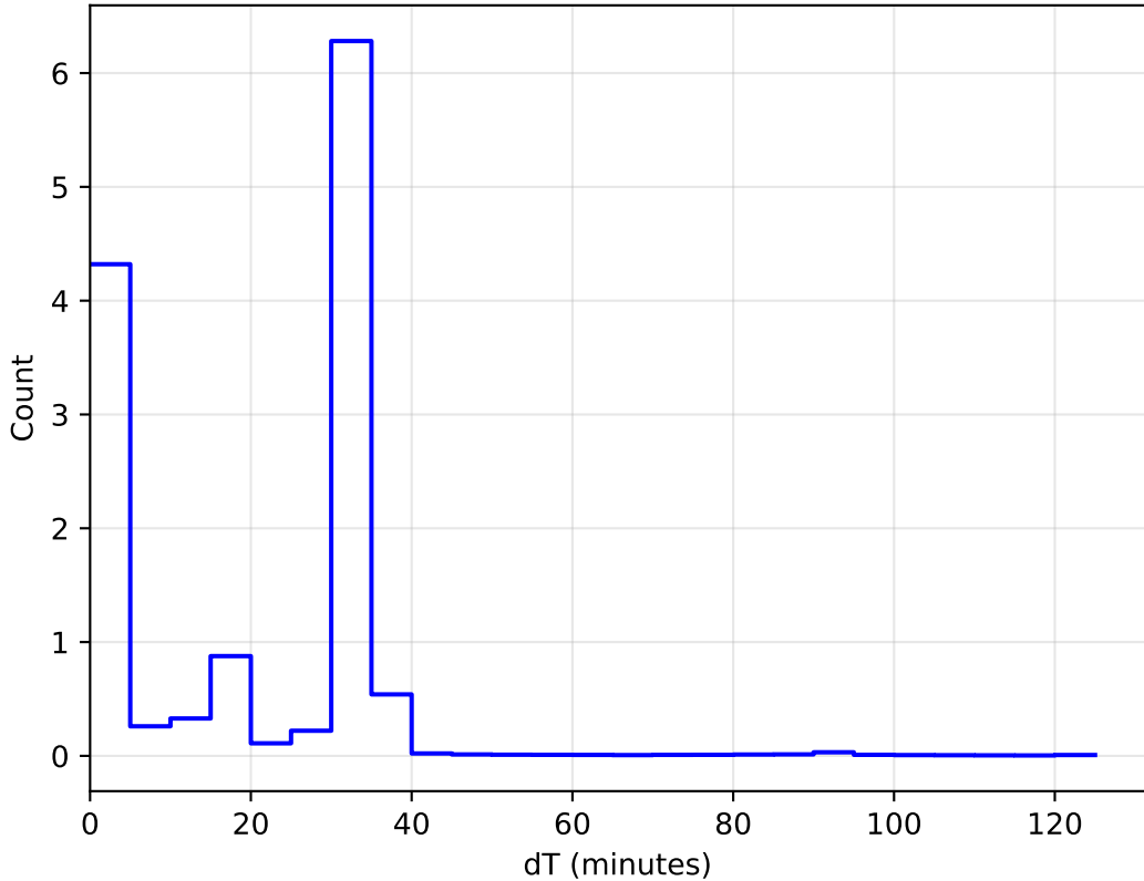
too_elab_r16_d3_ugrizy_v3.4_10yrs All sky: DeltaT Histogram 1e6
