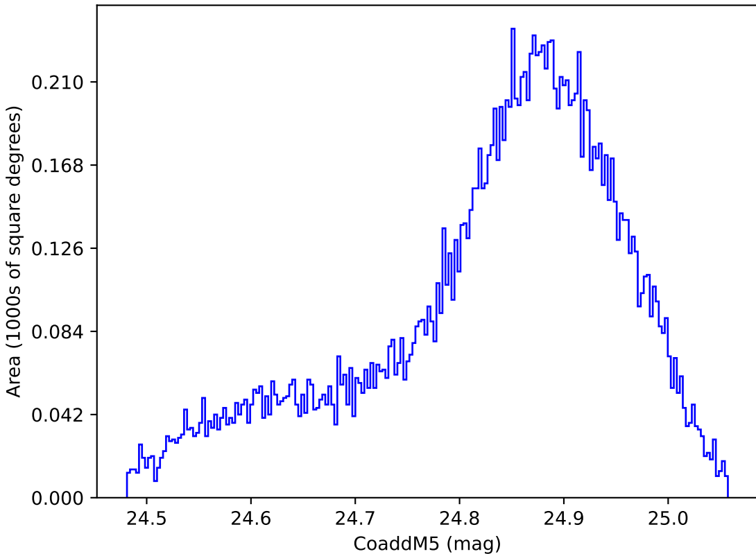
too_elab_r16_d3_ugrizy_v3.4_10yrs WFD y band: CoaddM5
