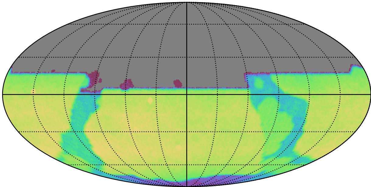
too_elab_r16_d3_ugrizy_v3.4_10yrs All sky y band: CoaddM5
