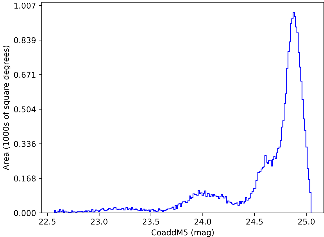
too_elab_r16_d3_ugrizy_v3.4_10yrs All sky y band: CoaddM5
