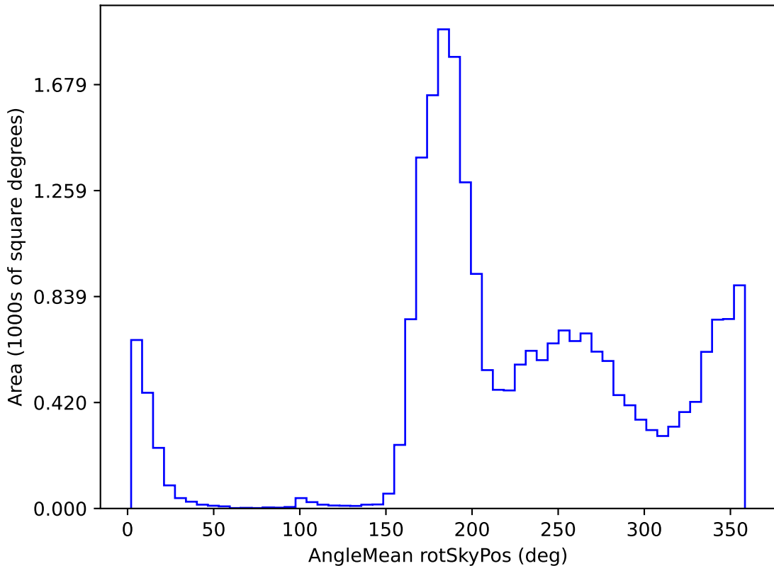
too_elab_r16_d3_ugrizy_v3.4_10yrs All sky y band: AngleMean rotSkyPos
