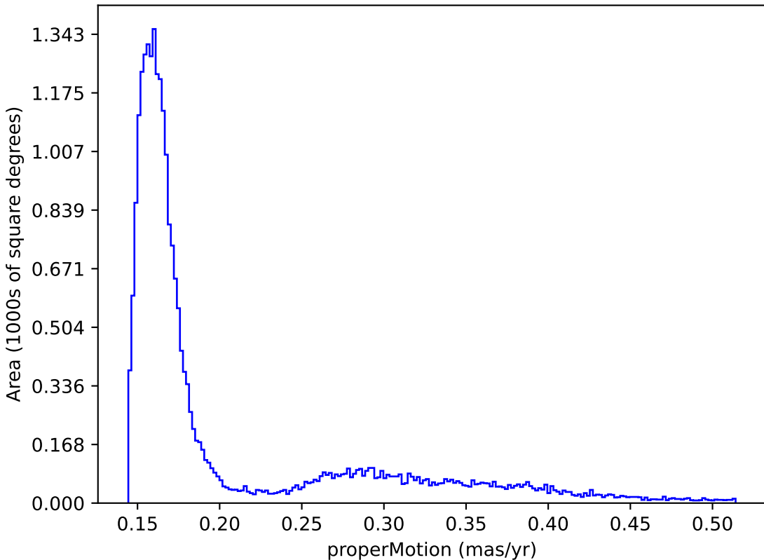
too_elab_r16_d3_ugrizy_v3.4_10yrs : properMotion
