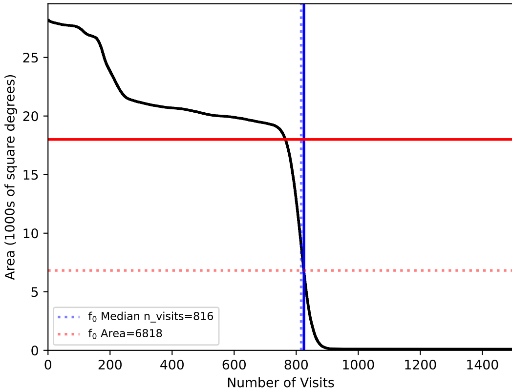
too_elab_r16_d3_ugrizy_v3.4_10yrs : f0
