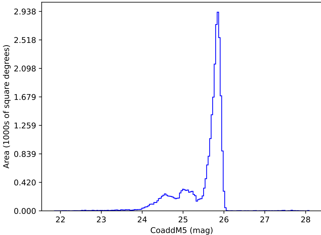
too_elab_r16_d3_ugrizy_v3.4_10yrs z: CoaddM5
