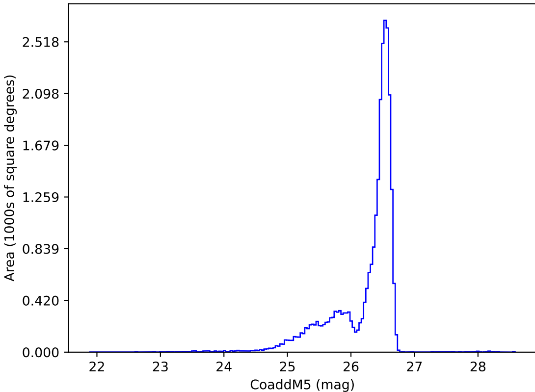
too_elab_r16_d3_ugrizy_v3.4_10yrs i: CoaddM5
