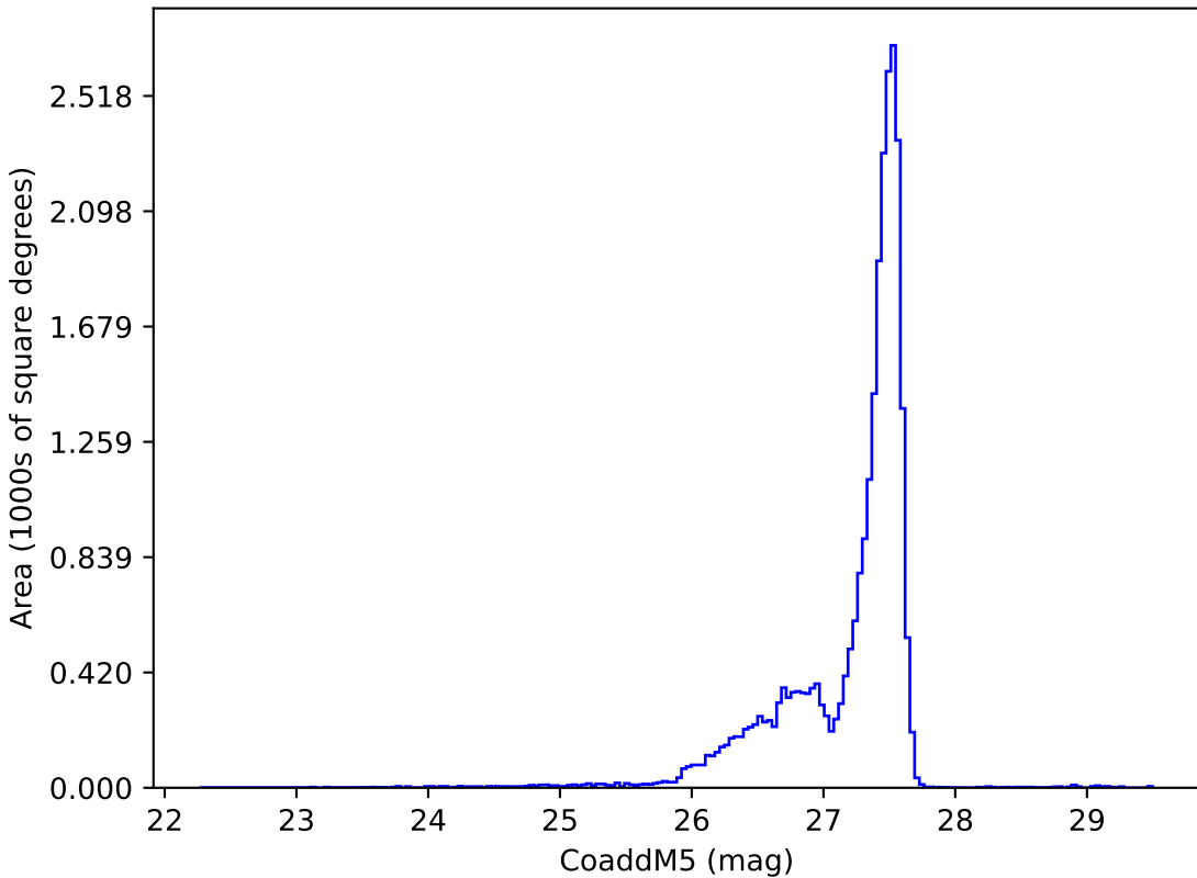
too_elab_r16_d3_ugrizy_v3.4_10yrs : CoaddM5
